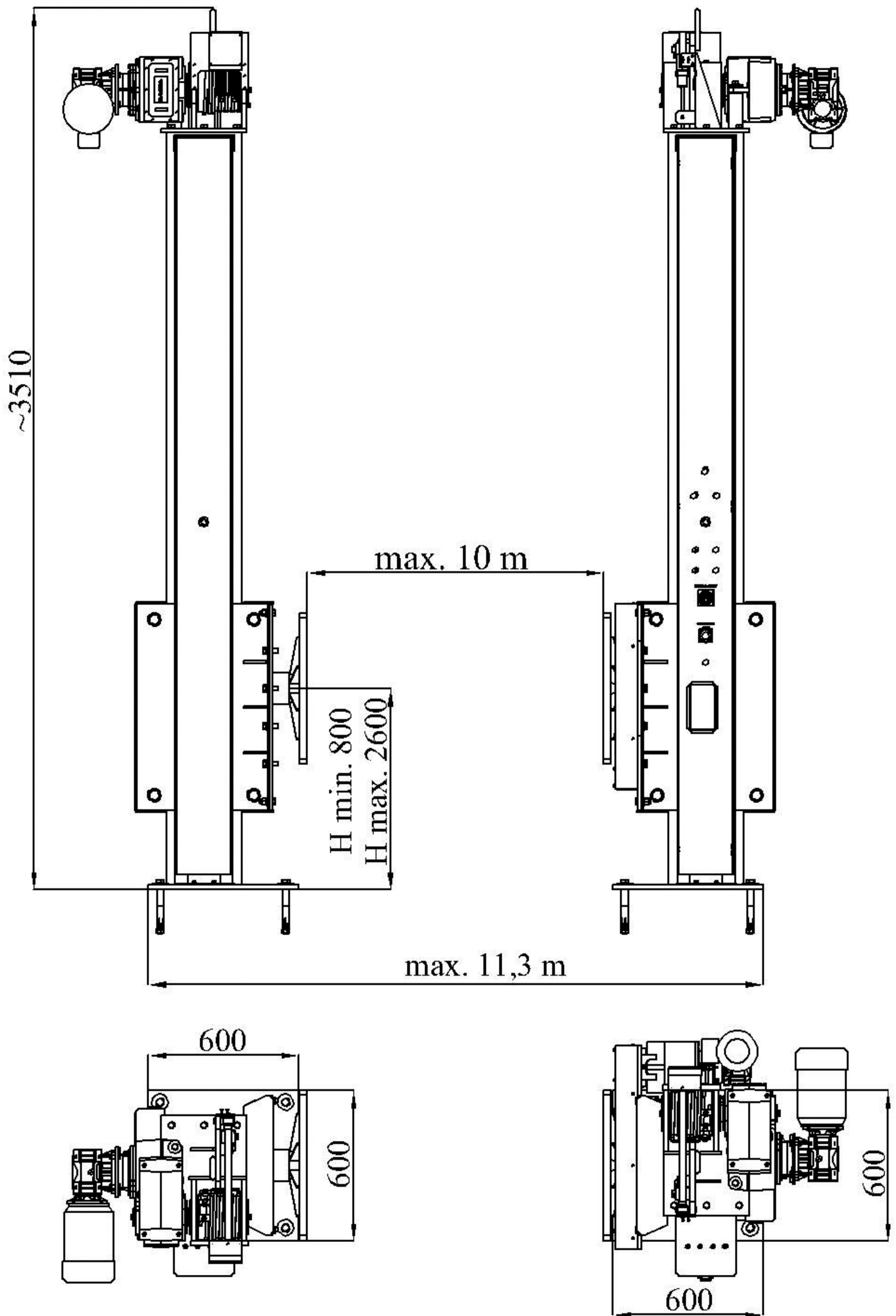
Rysunek gabarytowy Rys. 1
